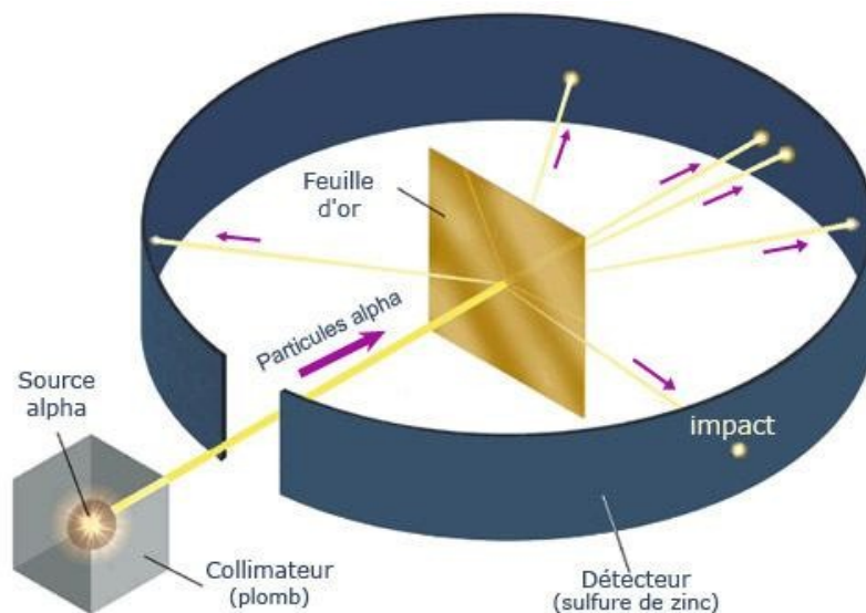
Figure 3: Dispositif expérimental de Rutherford
