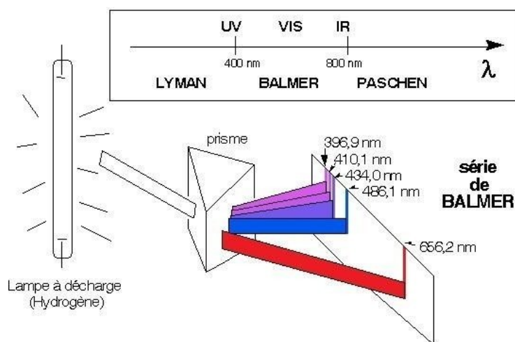
Figure 1. Spectre d'émission de l'atome d'hydrogène
